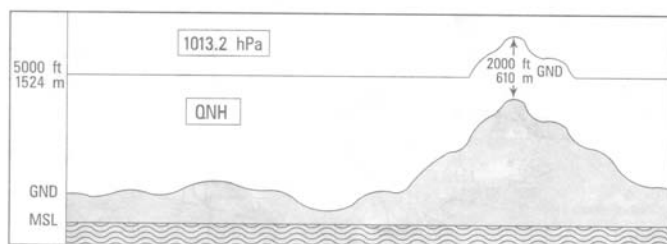
HÖHENMESSEREINSTELLUNG ALTIMETER SETTING
